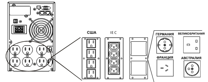
Рис. 1.5 Выходные разъемы
