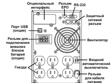
Рис. 1.1 700 ВА / 1 КВА / 1,5 КВА
