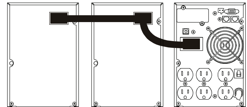
Рис. 2.2 Подключение внешних блоков батарей
