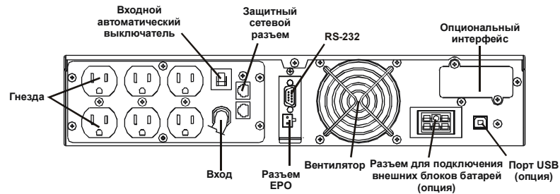
Рис. 1.3 700 ВА / 1 К / 1,5 КВА
