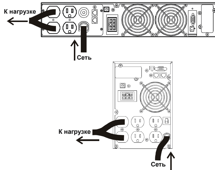
Рис. 2.1 Подключение на входе/выходе
