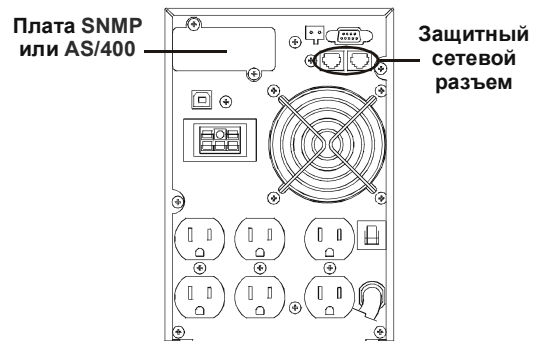
Рис. 2.5 Сетевые соединения
